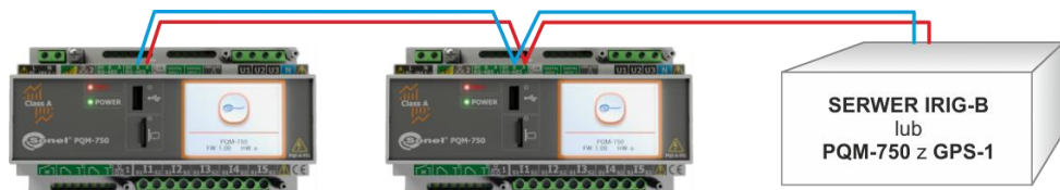
Rys. 32. Przykład sieci synchronizacyjnej IRIG-B
