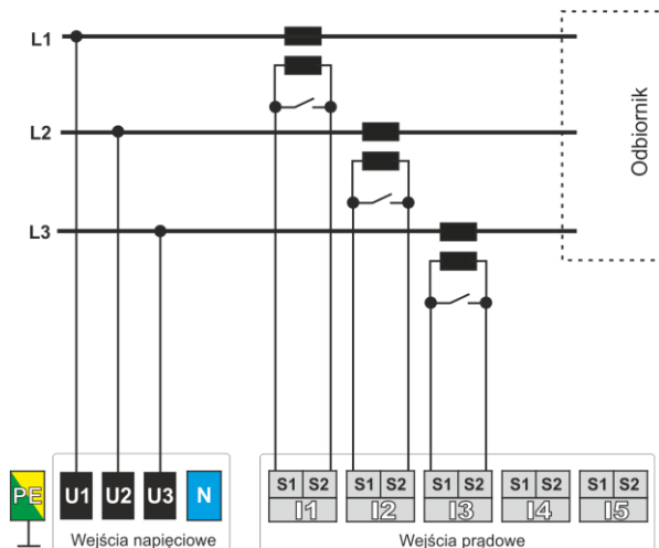
Rys. 28. Schemat podłączenia – układ 3-fazowy 3-przewodowy, bezpośrednie podłączenie napięć.
