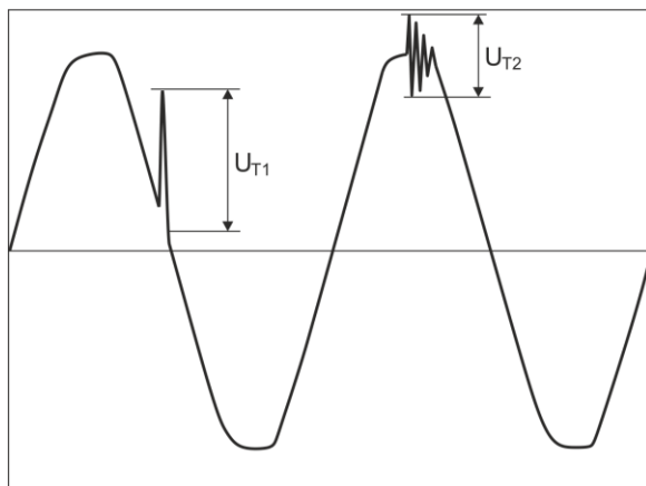
Rys. 36. Sposób wyznaczania amplitud transjentów.
