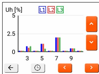
Rys. 14. Ekran harmonicznych napięć. Na każdym ekranie wyświetlonych jest 9 harmonicznych, a naciśnięcie strzałek góra i dół pozwala przechodzić do kolejnych lub poprzednich 9-ciu. Naciśnięcie strzałki w prawo powoduje przejście do harmonicznych prądów.
