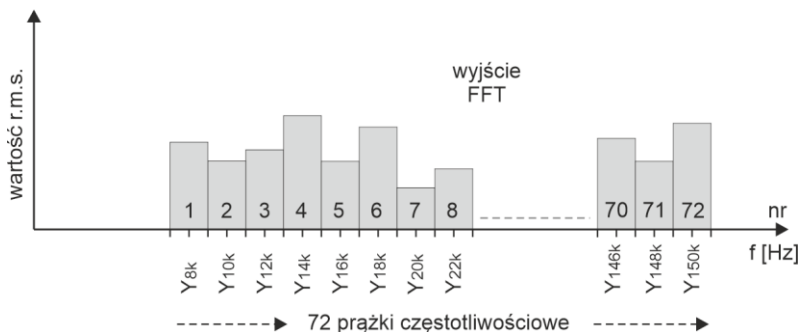
Rys. 35. Prążki częstotliwościowe w pomiarze pasma 9-150 kHz.
