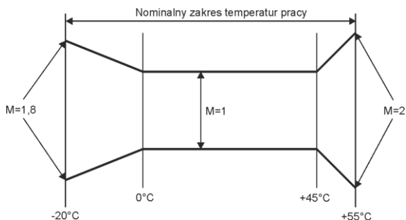
Rys. 37. Mnożnik odchyłki pomiarowej w zależności od temperatury otoczenia.
