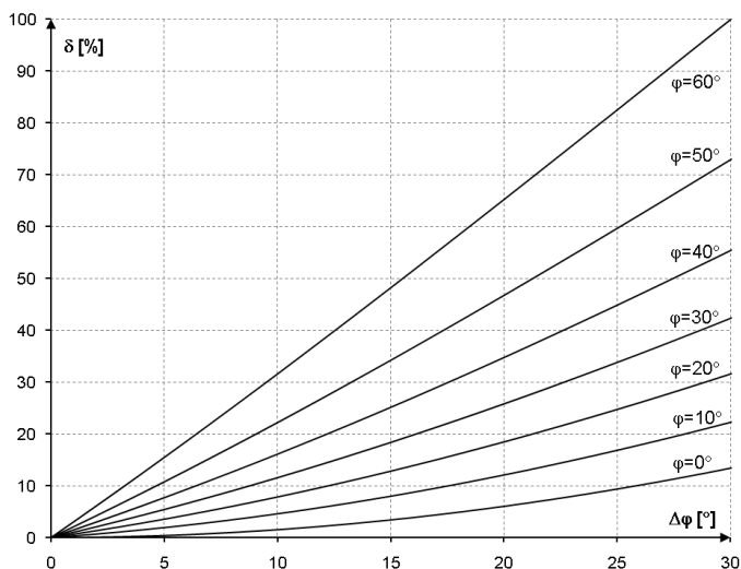
Rys. 38. Niepewność dodatkowa od błędu fazy w zależności od kąta przesunięcia fazowego.
