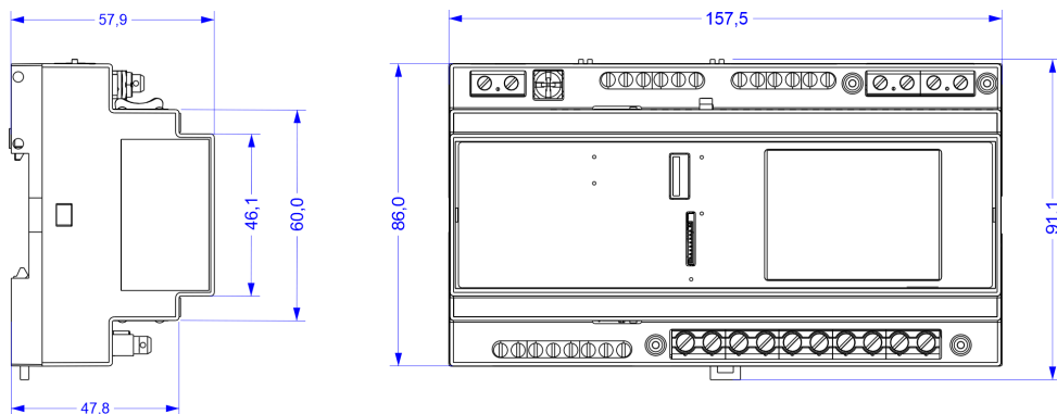
Rys. 4. Wymiary zewnętrzne analizatora (w milimetrach).
