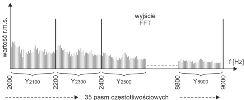
Rys. 34. Pomiar w paśmie częstotliwościowym 2-9 kHz.
