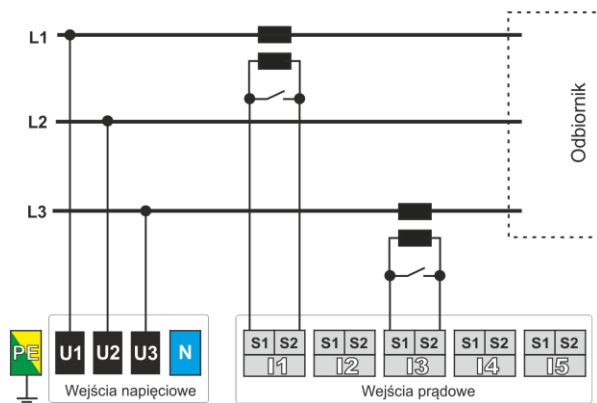
Rys. 29. Schemat podłączenia – układ 3-fazowy 3-przewodowy, metoda pomiarowa Arona.
