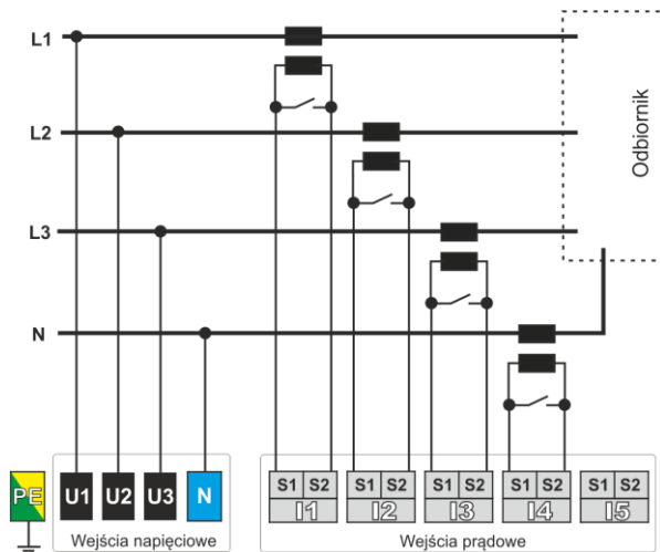
Rys. 27. Schemat podłączenia – układ 3-fazowy 4-przewodowy, bezpośrednie podłączenie napięć.
