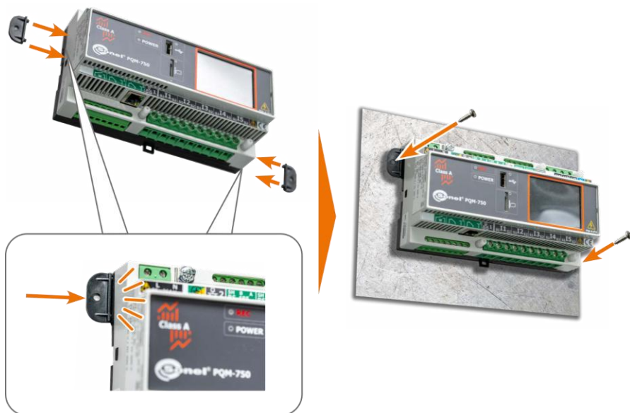
Rys. 6. Montaż analizatora do ściany przy użyciu dostarczonych uchwytów.
