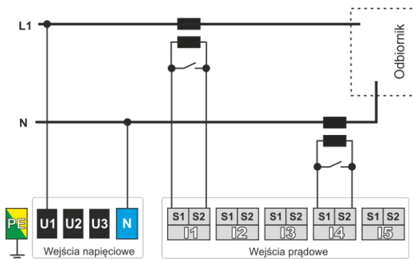
Rys. 25. Schemat podłączenia – układ jednofazowy, bezpośrednie podłączenie napięć.
