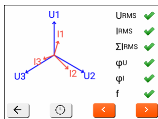
Rys. 11. Wykres wskazowy ze wskaźnikami poprawności podłączenia.
