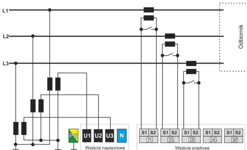
Rys. 30. Schemat podłączenia – układ 3-fazowy 3-przewodowy pośredni z przekładnikami napięciowymi.
